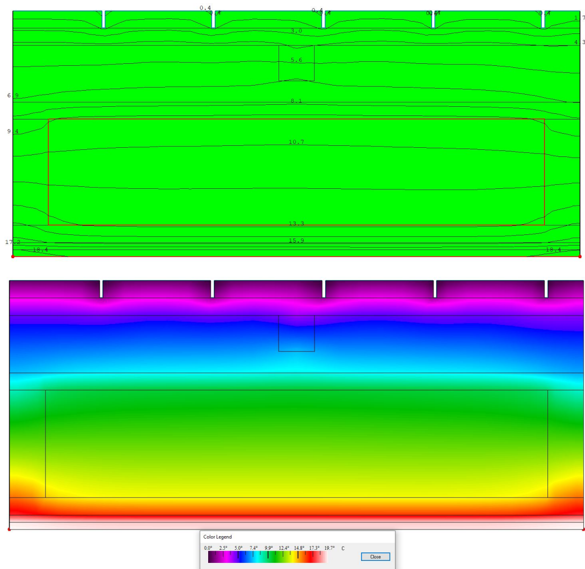
3.51. ábra Borított gerendafűdém (A1) thermografikus elemzése (saját ábra)
