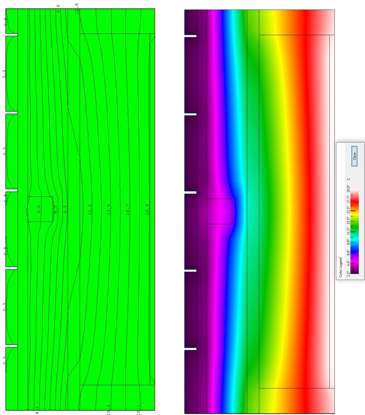
3.45. ábra Módosított pórfödém (P1*) thermografikus elemzése (saját ábra)
