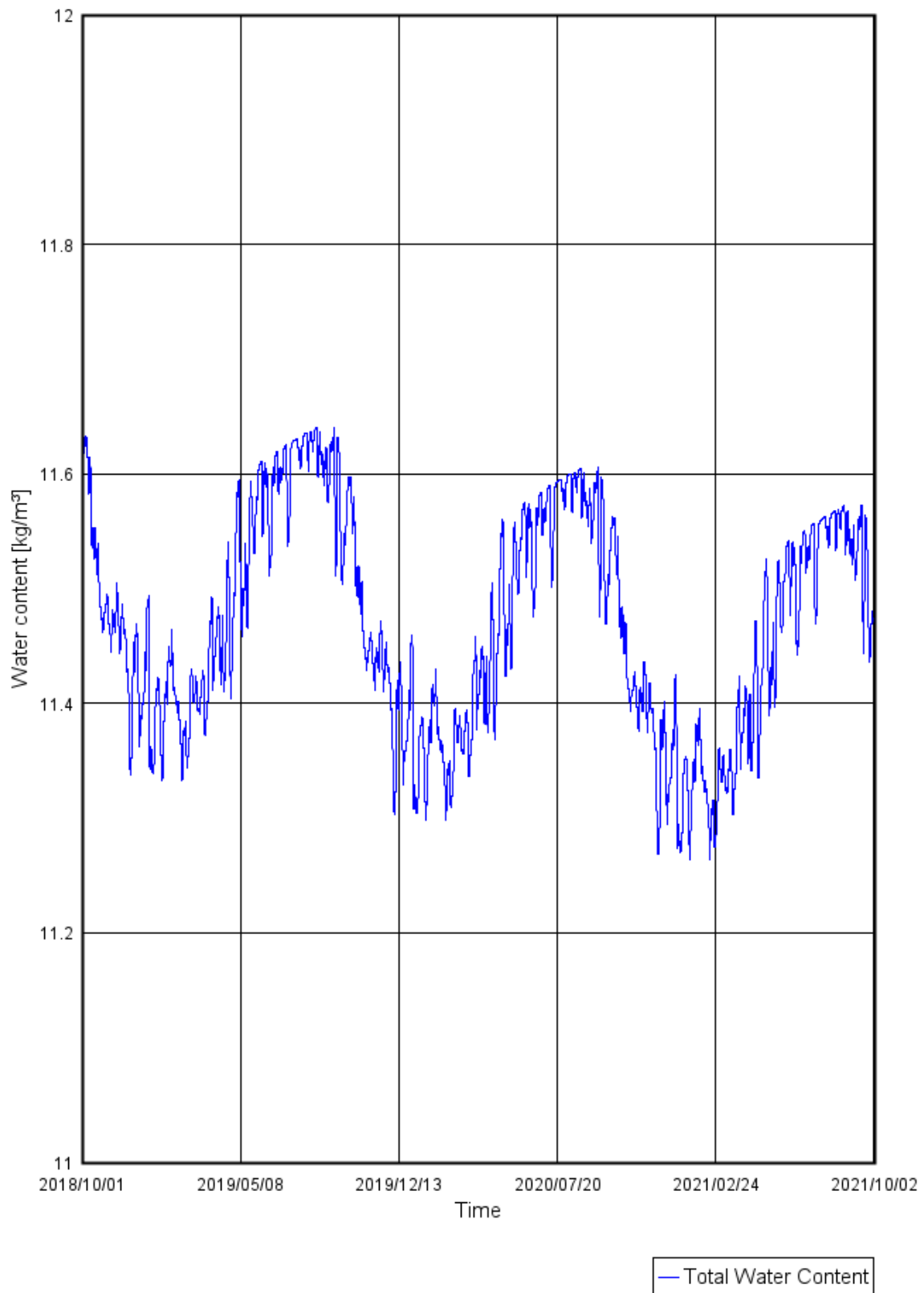
3.94. ábra Xd-típusú fűdémszerkezet teljes víztartalmának elemzése 3 éves ciklusban (idő-víztartalom függvényében, saját ábra)
