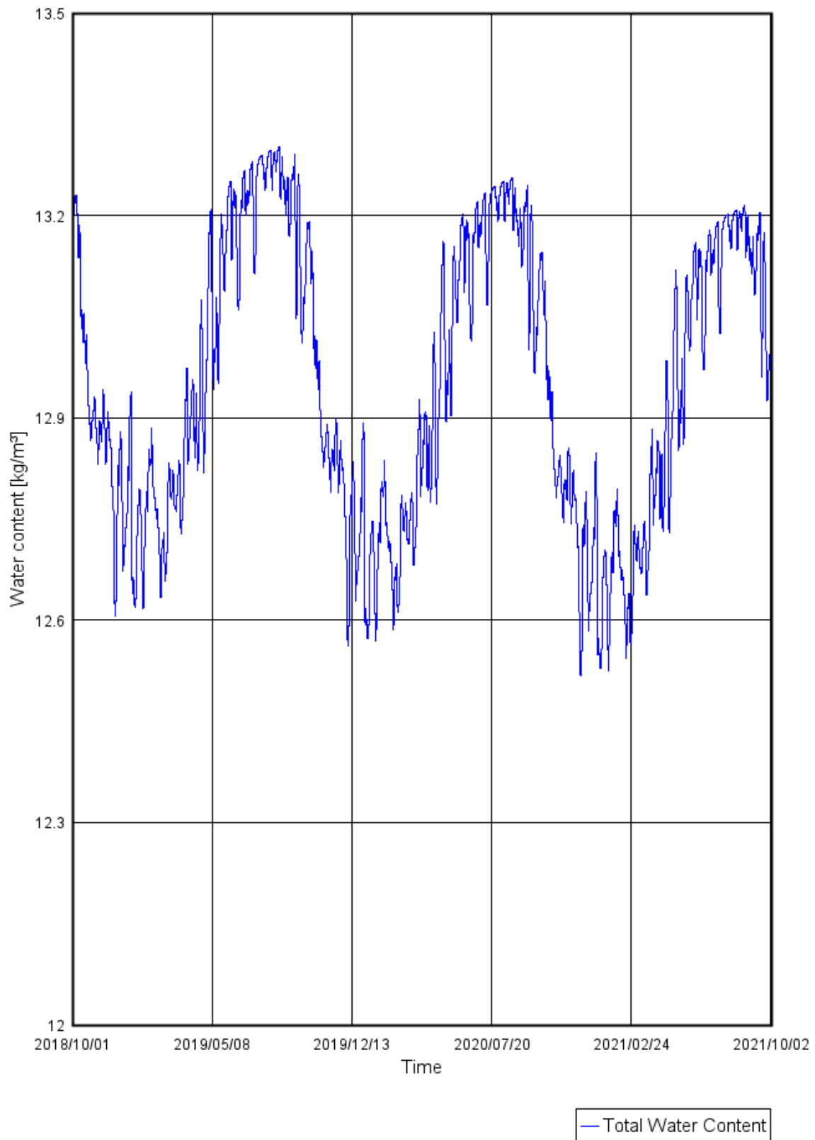
3.82. ábra Pallógerendás poroszsüveges fafödém (Xa) teljes víztartalma 3 éves ciklusban (saját ábra)
