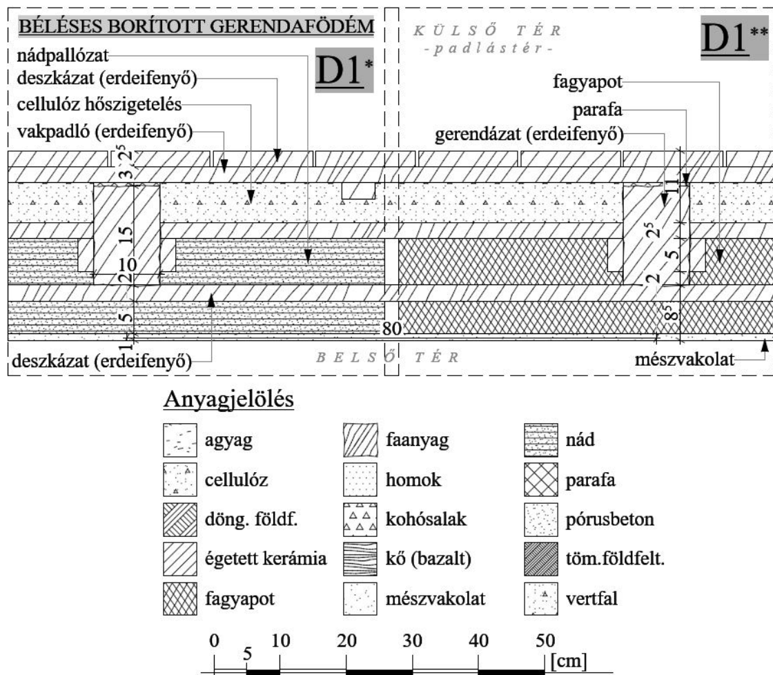
3.57. ábra Módosított béléses borított gerendafödém (D1*, D1**) metszete (saját ábra)
