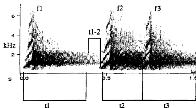
17. ábra: A fűrjkakas hangjának szonogramja COLLINS & GOLDSMITH (1998) nyomán. A t1 , t2 , t3 – a szótagok hossza; f1 , f2 , f3 – a szótagok fundamentális frekvenciája; t1-2 – az első két szótag közötti intervallum
