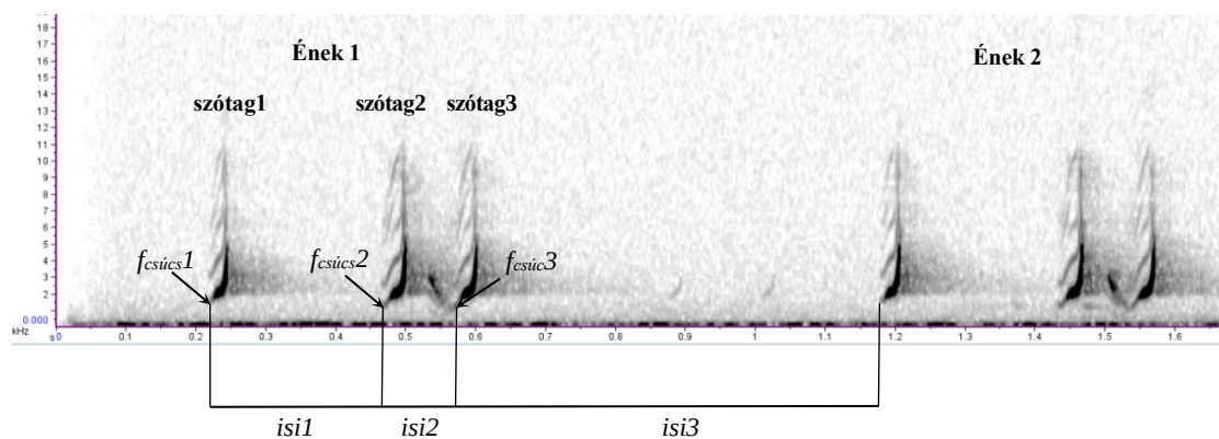
18. ábra: Fűrjkakas énekének szonogramja a MOSON Project területén készített felvétel alapján ( isi1 – az 1. és 2. szótagok közt eltelt idő; isi2 – a 2. és 3. szótagok közt eltelt idő; isi3 – a 3. és 1. szótagok közt eltelt idő; f_{csúcs1-3} – az 1-3. szótagok csúcsfrekvenciái)
