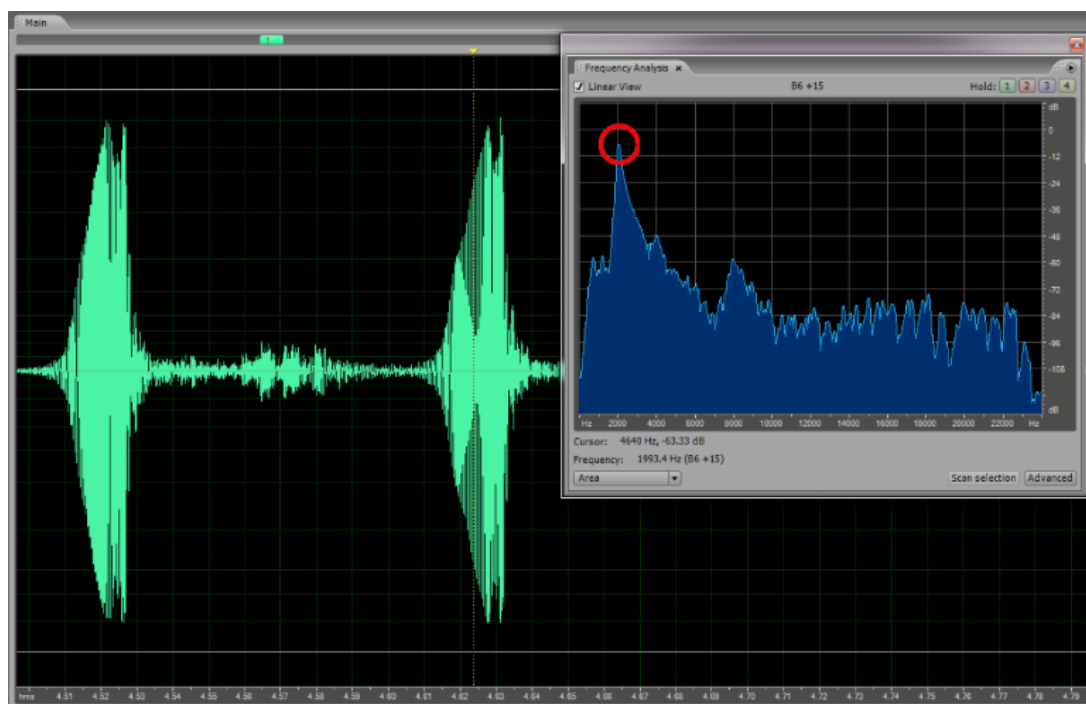
19. ábra: A fundamentális frekvencia mérése a fűj hangok szótagjain – Adobe Audition 3.0
