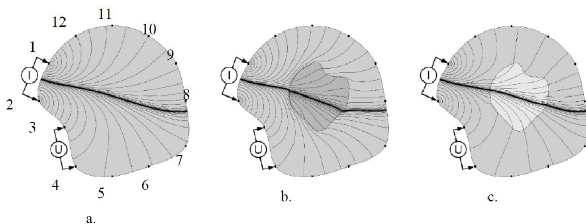
15. ábra: Picus Treetriconic műszer működési elve (forrás: Treetriconic manual eng 2011_03, argus electronic gmbh, Vízvári 2015)
