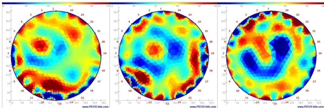
31. ábra: a 152-es erőrészlet 1-es mintájának eredményei
