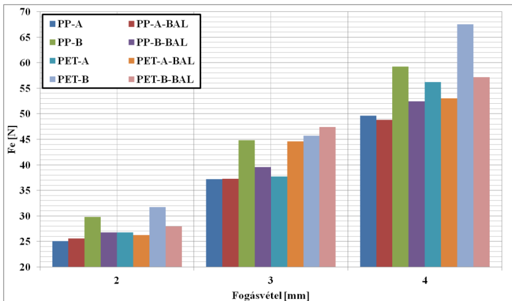
IV.29. ábra. Az eredő erő a fogásvétel függvényében különböző élelhelyezési szögekkel
