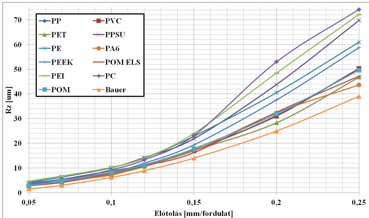
IV.2. ábra. Az egyenetlenség magasság változása a fordulatonkénti előtolás növelésével
