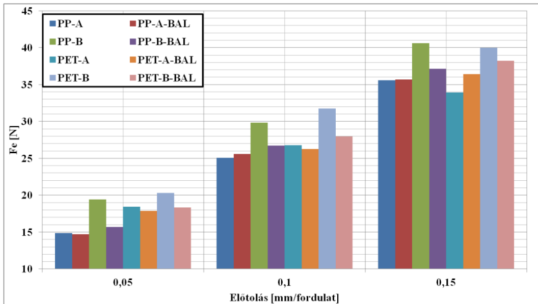
IV.28. ábra. Az eredő erő az előtolás függvényében különböző élelhelyezési szögekkel
