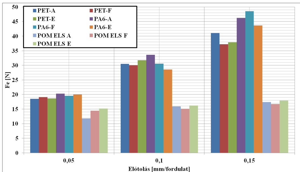
IV.25. ábra. Különböző gyártmányú lapkával való esztergálás közben mért forgácsoló erők
