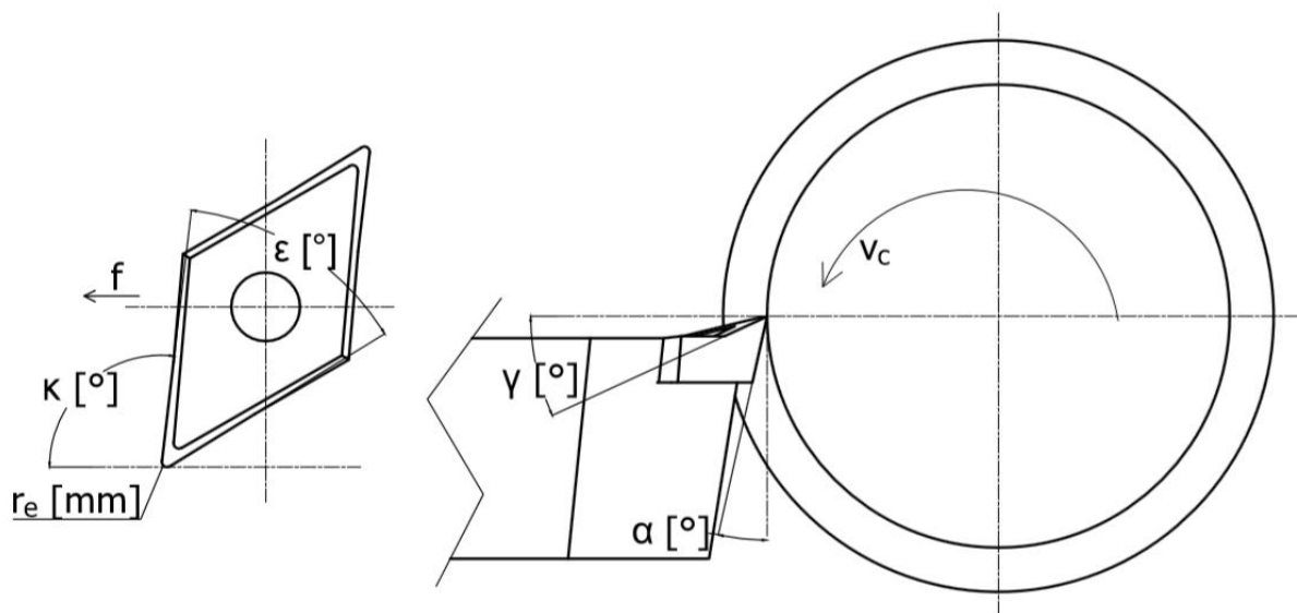
II.9. ábra. Jellemző szerszámgeometriai paraméterek
