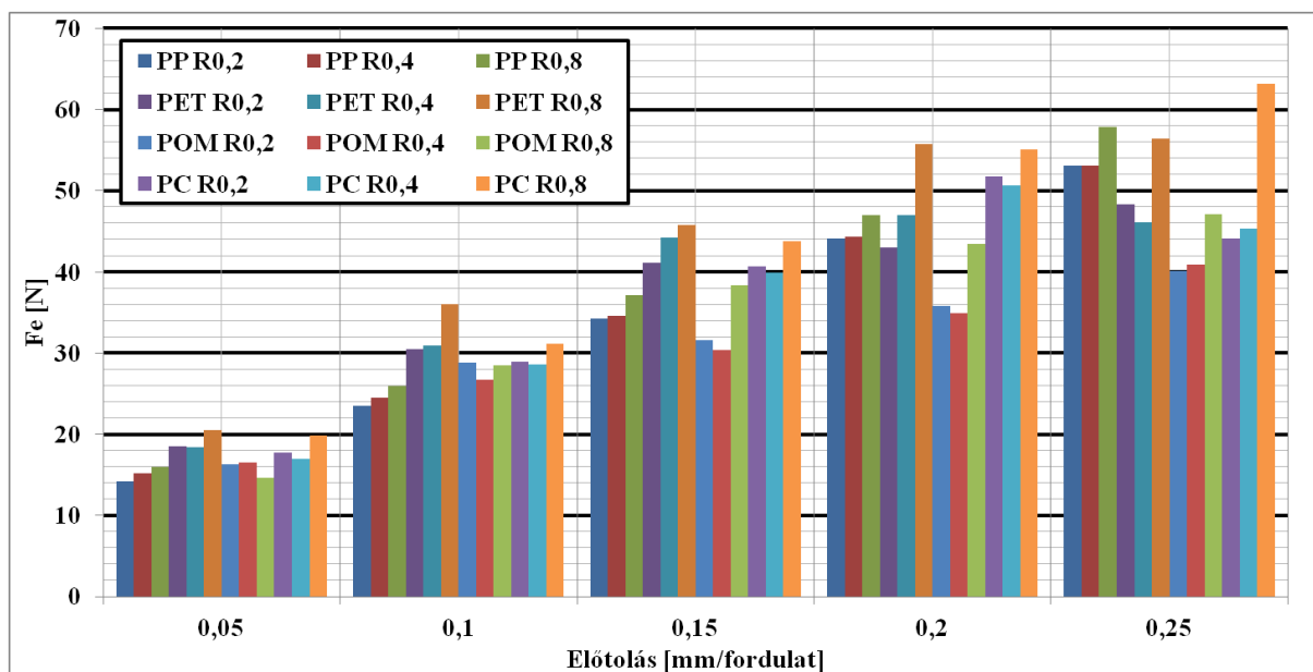
IV.22. ábra. A forgácsolóerő változása különböző csúcsráduszu lapkák esetén
