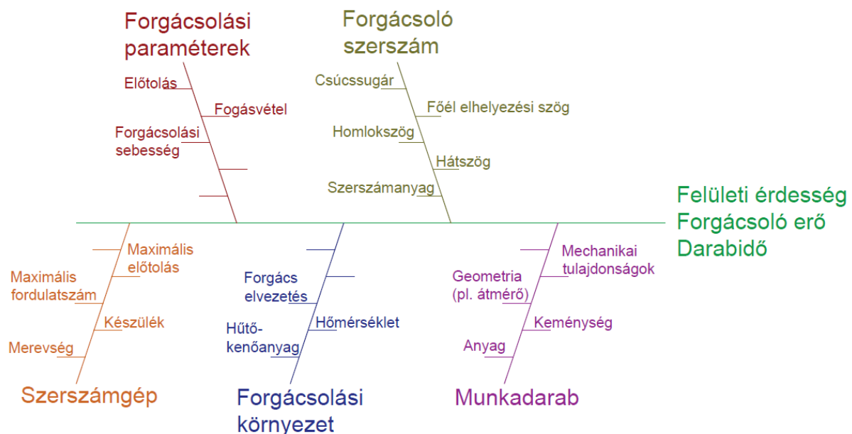
II.1. ábra. A forgácsolási folyamatot bemutató Ishikawa diagram
