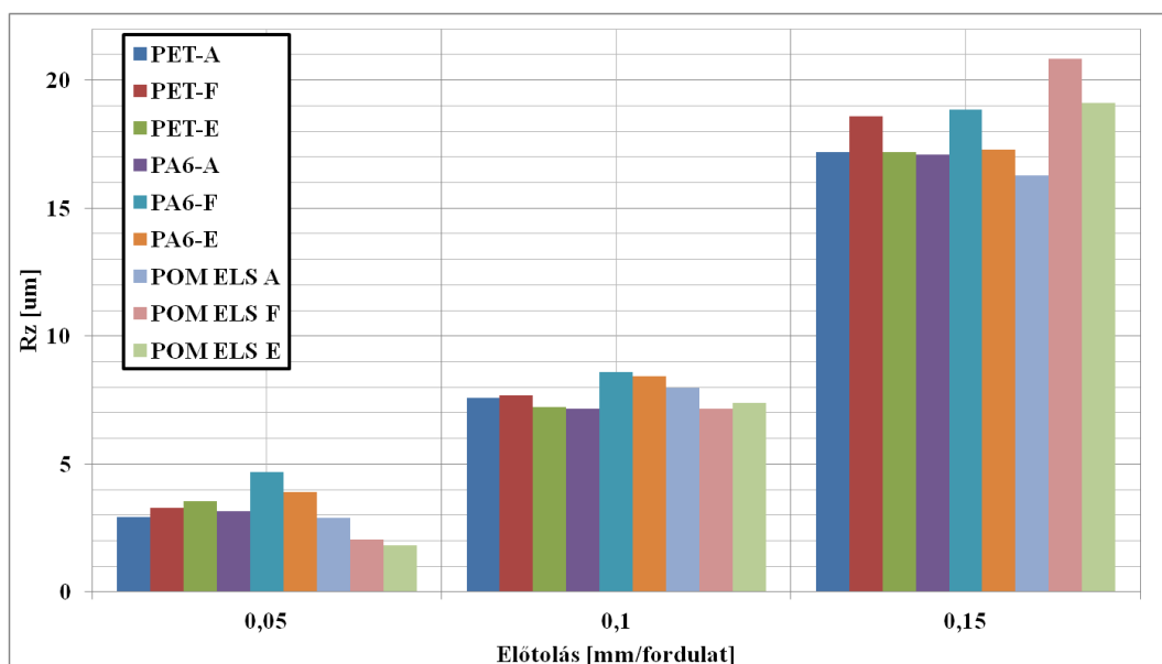
IV.24. ábra. Különböző lapkával forgácsolt próbatestek felületi minősége
