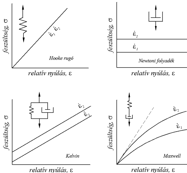
17. ábra. A legegyszerűbb rheológiai modellek és azok jelleggörbéi (SITKEI, 1981)
