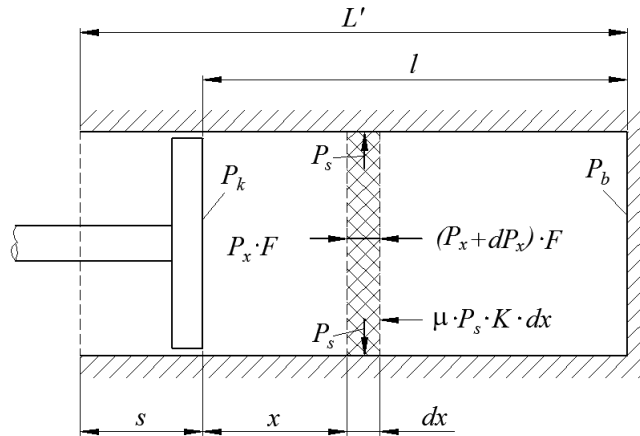
27. ábra. A tömörítő henger nyomásviszonyai (SITKEI, 1981)
