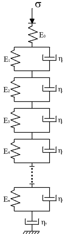
21. ábra. Az általánosított Kelvin-modell (FINDLEY, 1976)
