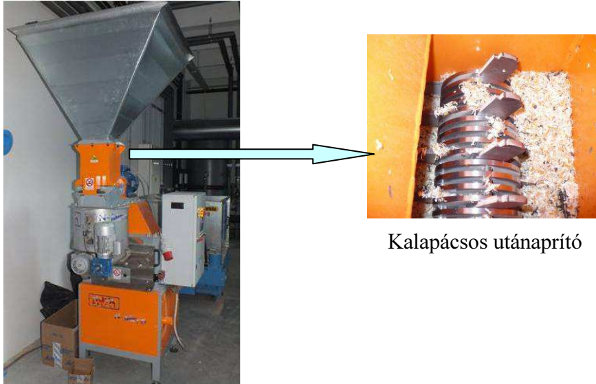
34. ábra. NOVA PELLET N-MICRO B típusú pelletáló gép (maximális kapacitása folyamatos alapanyag adagolás mellett: 200 kg/óra)
