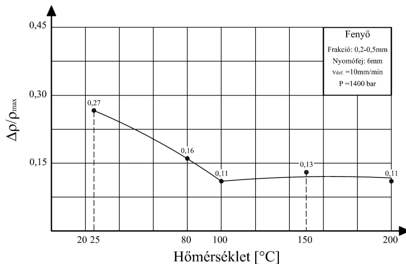
69. ábra. A relatív sűrűségcsökkenés a hőmérséklet függvényében fenyő mintánál 1400 bar nyomáson
