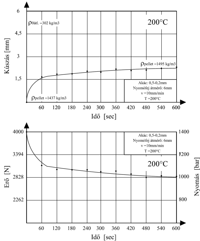
86. ábra. Akácminta relaxációs és becsült kúszási görbéje az idő függvényében 1400 bar nyomáson, 200^\circ\text{C} vizsgálati hőmérsékleten
