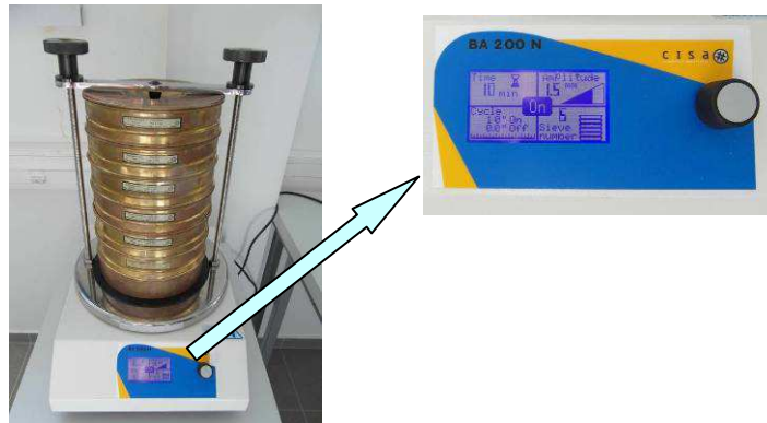
35. ábra. CISA BA 200 N típusú elektromágneses digitális szitázó készülék
