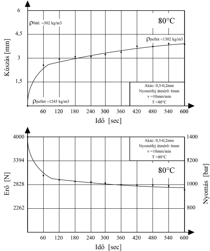
85. ábra. Akác minta relaxációs és becült kúszási görbéje az idő függvényében 1400 bar nyomáson, 80^\circ\text{C} vizsgálati hőmérsékleten
