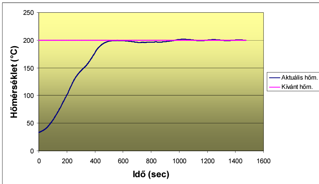
48. ábra. Hőmérsékletfelfutási görbe hőntartással 200^{\circ}\text{C} állandó hőmérsékletig
