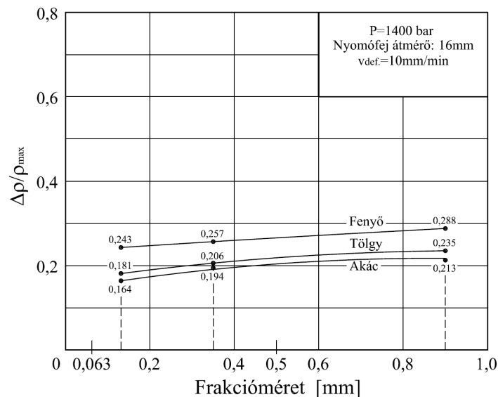
91. ábra. A kirugózás okozta relatív sűrűség változása a frakcióméret függvényében
