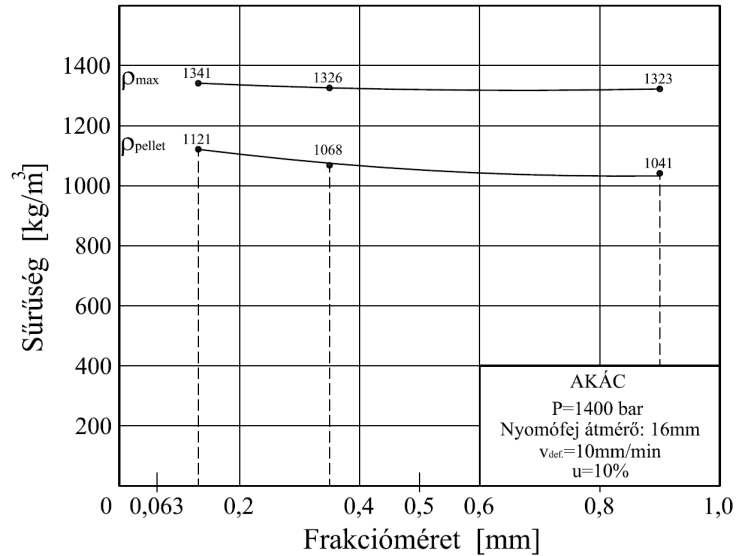
90. ábra. A pellet sűrűség változása a frakcióméret függvényében akác mintánál 16 mm-es nyomófej átmérőnél
