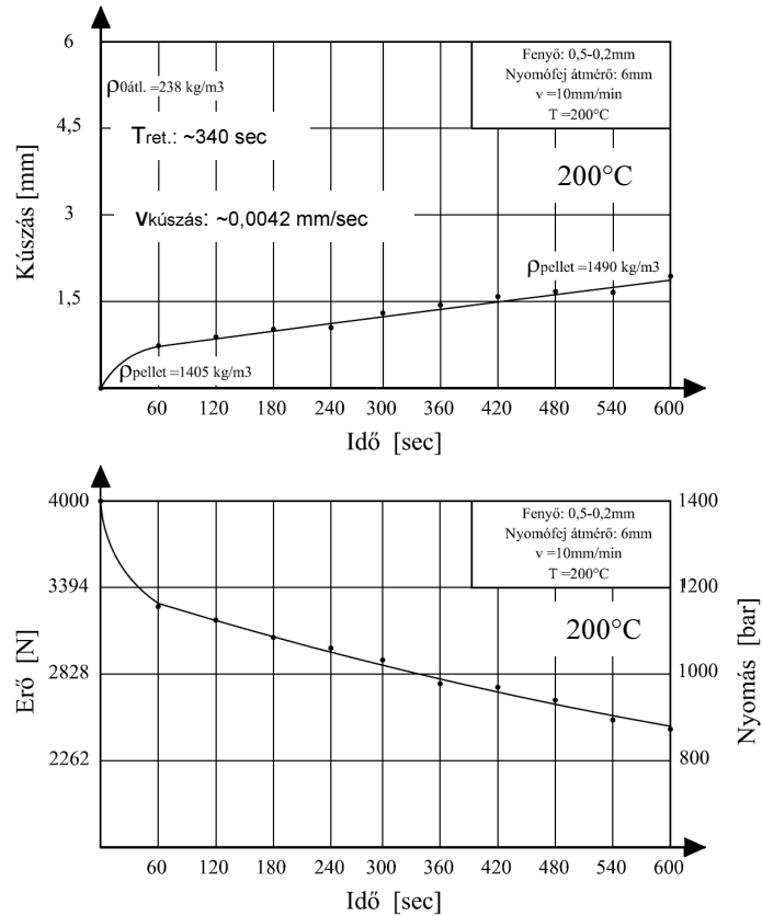
84. ábra. Fenyő minta relaxációs és becült kúszási görbéje az idő függvényében 1400 bar nyomáson, 200^\circ\text{C} vizsgálati hőmérsékleten
