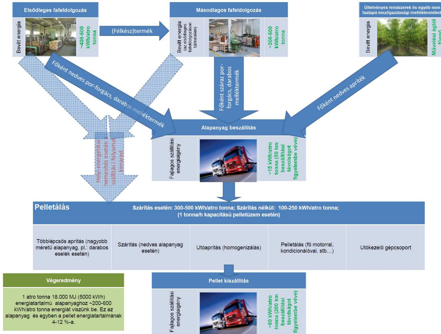
9. ábra. Magyarországi 1 tonna/óra kapacitású pelletgyártásra jellemző általános logisztika folyamatára (NÉMETH et al., 2012)
