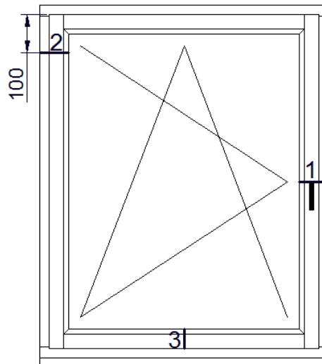
38. ábra A résméreték mérési pontjainak helyzete a kerület mentén
