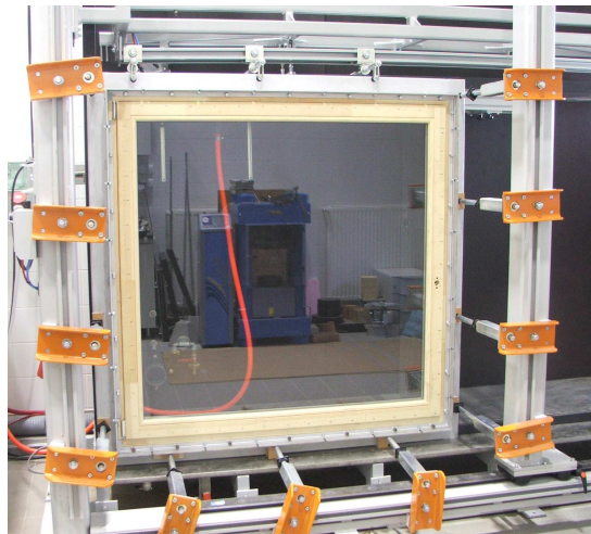
29. ábra A 11. számú próbatestet légzárási vizsgálat
