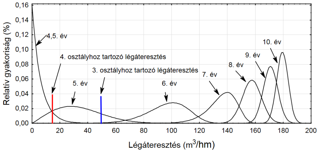
70. ábra A vizsgált nyílászáró 1 igénybevételi szintjéhez tartozó légzárási sűrűség-függvények
