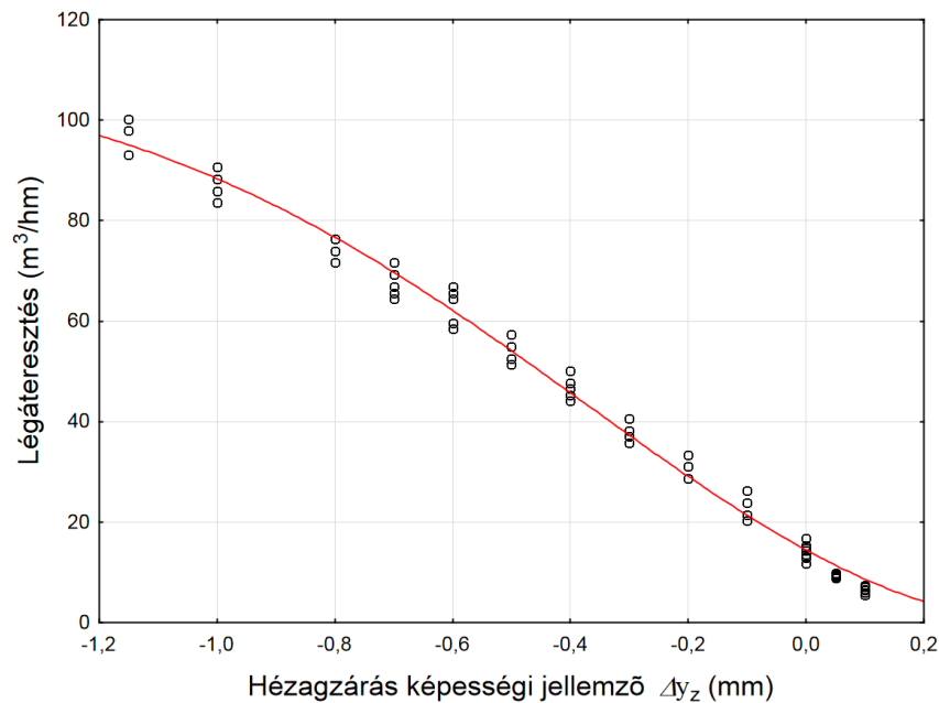
65. ábra Légáteresztés a hézagzárási mutató függvényében
