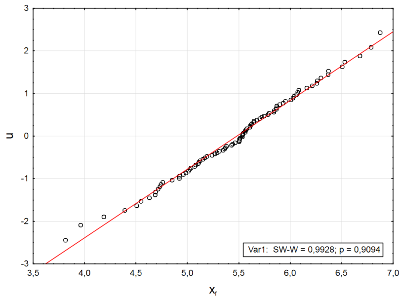
40. ábra Az adatok ábrázolása Gauss-hálón
