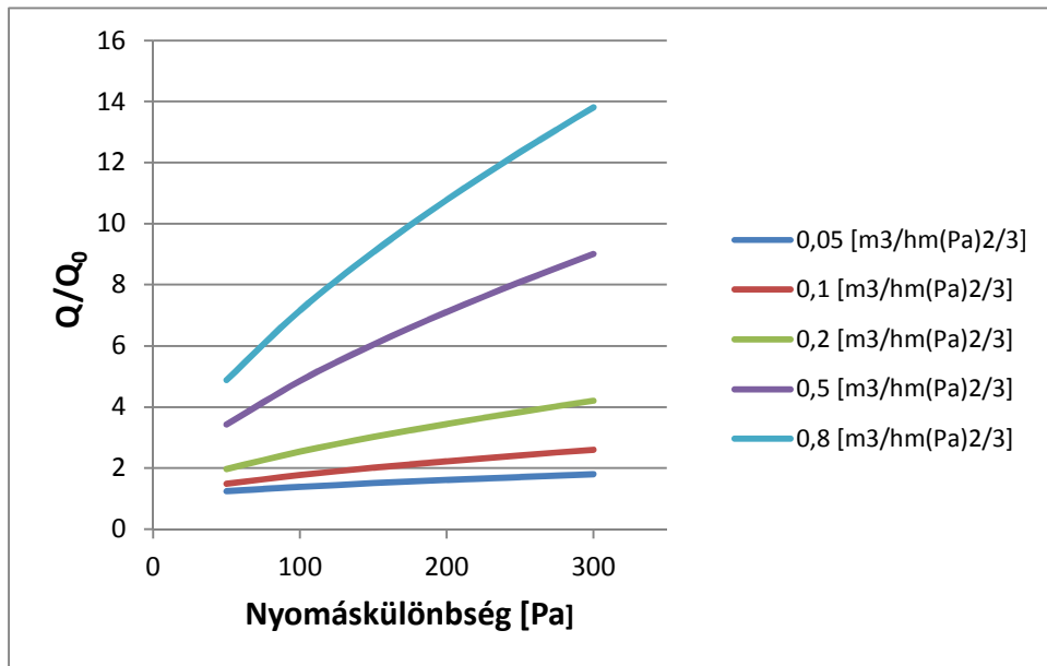
4. ábra A hővesztés a torlónyomás függvényében
