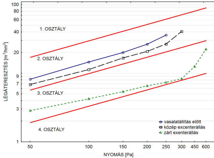
27. ábra A 7. számú próbatest osztályozó diagramja
