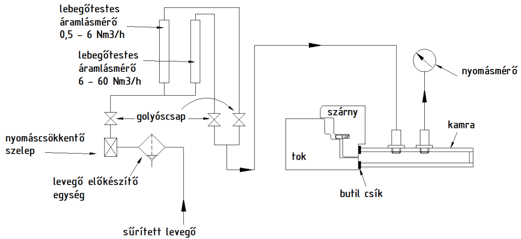
61. ábra A résáramlás meghatározásához használt mérőberendezés elvi vázlata
