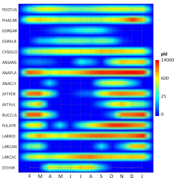
5.103. ábra: A gyakori vízimadár-fajok fenológiája a Balaton déli partján (2003–2008)
