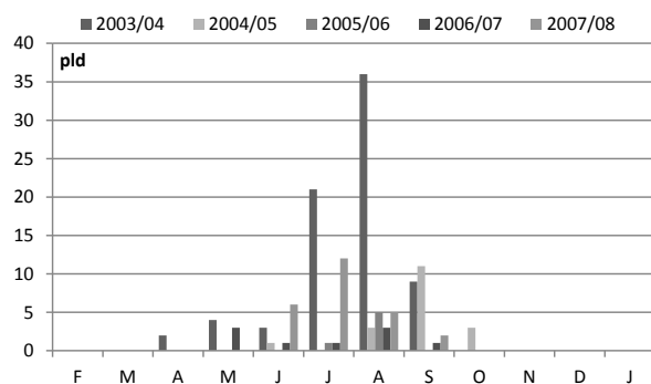
5.15. ábra: Havonkénti kis kócsag összegyedszám az egyes években
