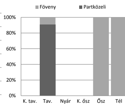
5.48. ábra: A kanalas réce aspektusonkénti élőhelyhasználat
