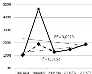
5.50. ábra: A barátréce populációváltozás indexe
