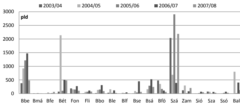
5.65. ábra: A kerceréce diszperziója az összegyedszámok alapján az egyes években
