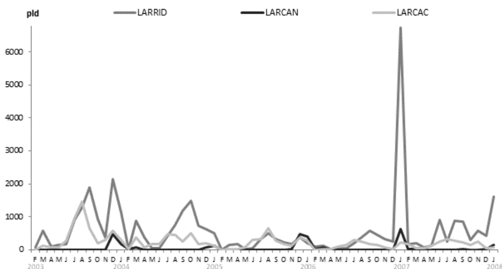
6.4. ábra: A három gyakori sirályfaj (dankasirály, vihasirály, sárgalábú/sztyeppi sirály) dinamikája az egyes hónapokban a Balaton déli partján (2003–2008)
