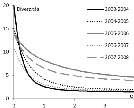
5.131. ábra: Az egyes évek diverzitási profiljai Balatonfenyvesnél
