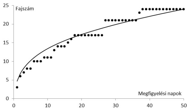
5.225. ábra: Fajtelítődési (rarefaction) görbe Siófoknál (2003–2008)
