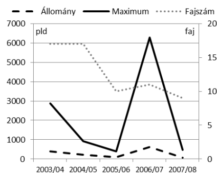
5.230. ábra: Vízimadarak átlagos állománynagysága, maximuma és fajszáma Balatonszabadinál az egyes években
