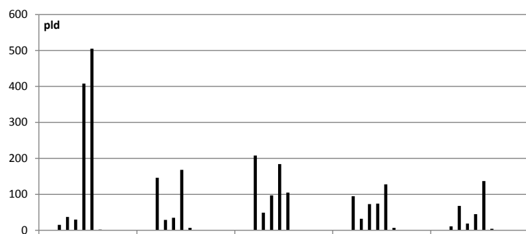
5.91. ábra: Küszvágó csér összegyedszám az egyes megfigyelési napokon (2003–2008)
