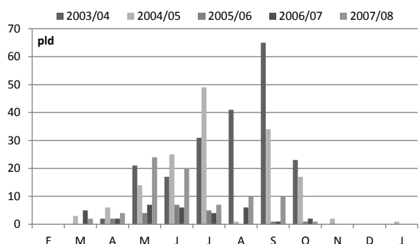
5.21. ábra: Havonkénti nagy kócsag összegyedszám az egyes években
