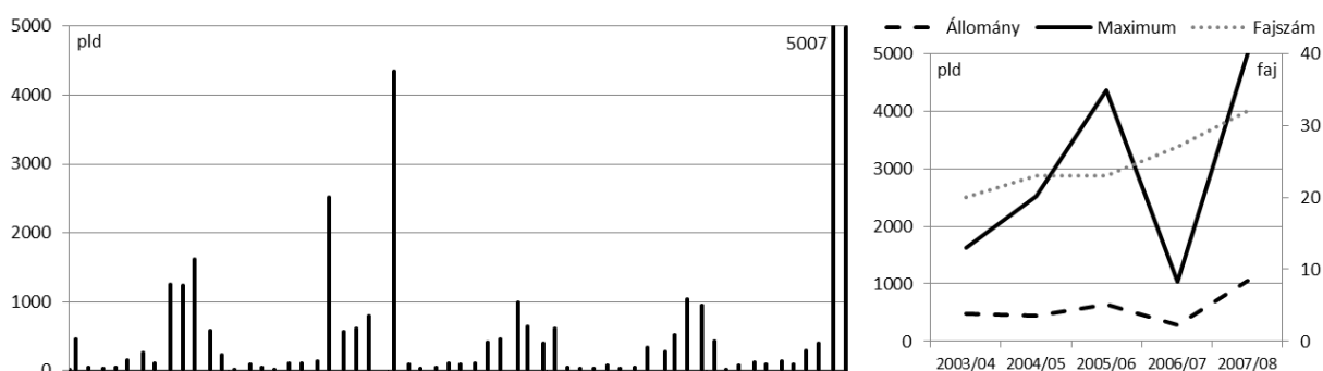
5.205. ábra: Vízmadarak összegyedszáma az egyes megfigyelési napokon Szántódnál (2003–2008)
