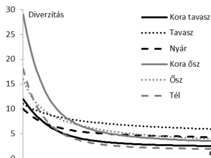
5.188. ábra: Az egyes aspektusok diverzitási profiljai Balatonszemesnél (2003–2008)
