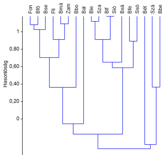
5.262. ábra: Vízimadarak partközeli és pattól távoli élőhelyhasználatának összehasonlítása ( \chi^2 -teszt) a délbaltóni partszakaszok szerint (2003–2008)
