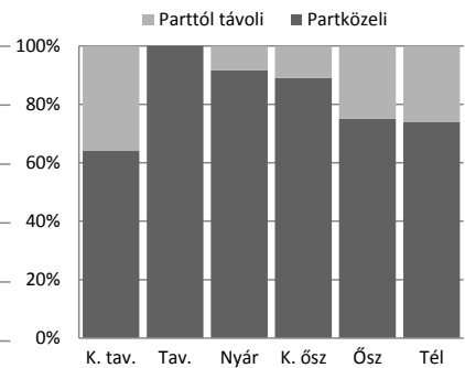
5.72. ábra: A szárcsa aspektusonkénti élőhelyhasználat
