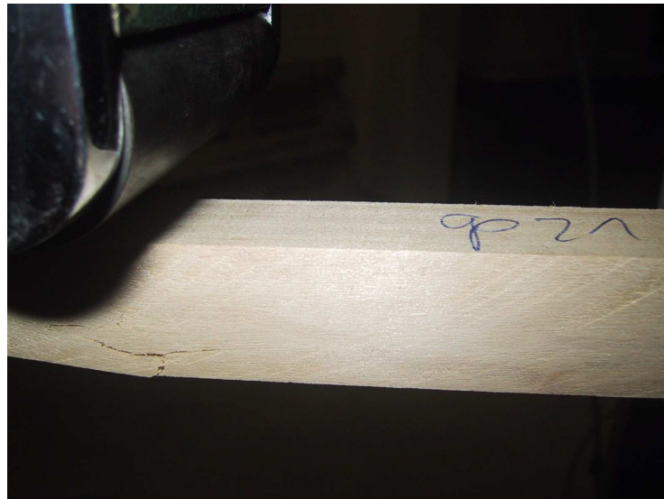
13. ábra: Rideg törés (FOTÓ: KATONA)
