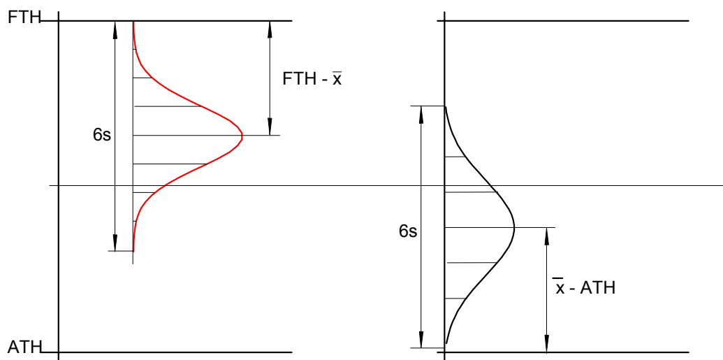
12. ábra: A képességi mutatók értelmezése
