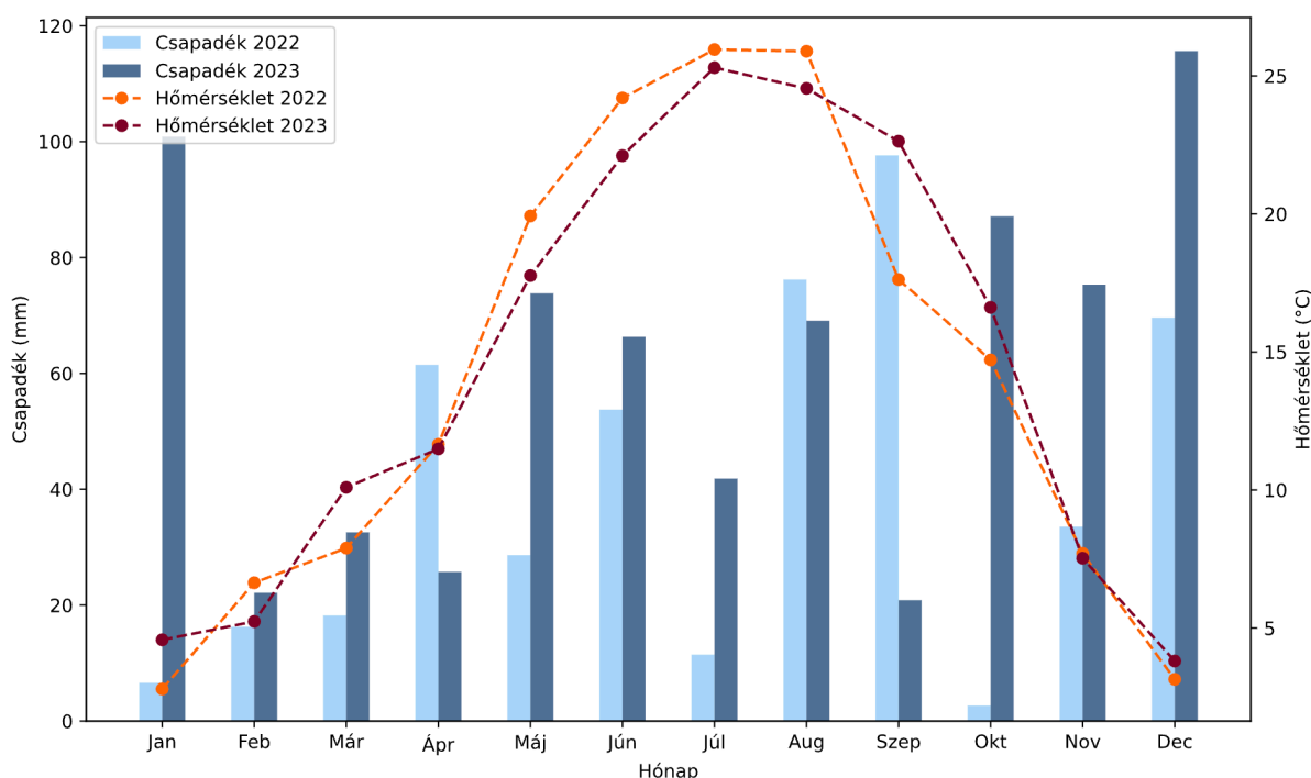
11. ábra: A bajnai agrárerdészeti terület átlagos hőmérséklet- és csapadékadatai a 2022-es és a 2023-as évben (a FORESEE adatbázis értékei alapján [URL15])
