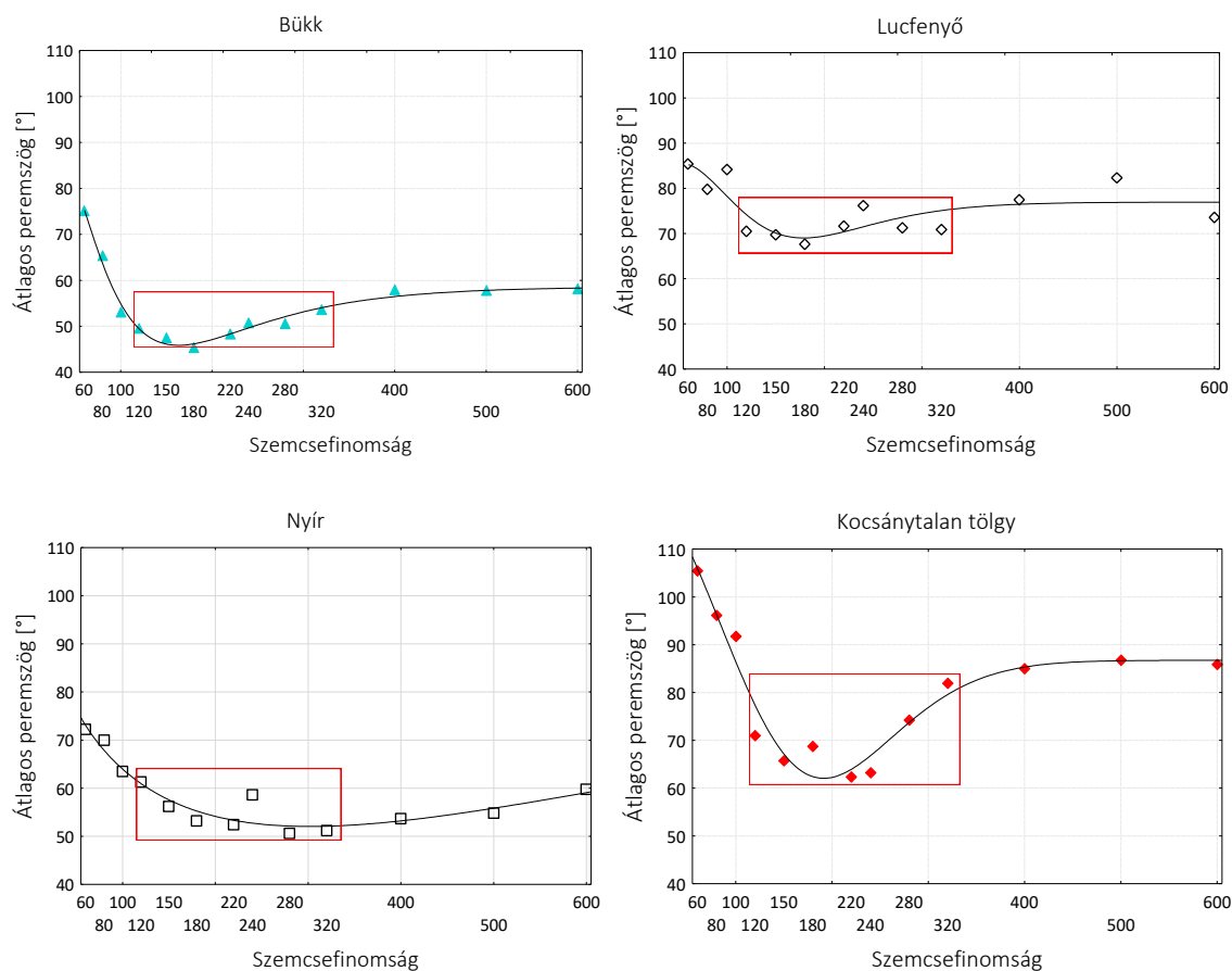
10. ábra Csizolt fafelületek átlagos peremszög értékei a szemcsefinomság függvényében
