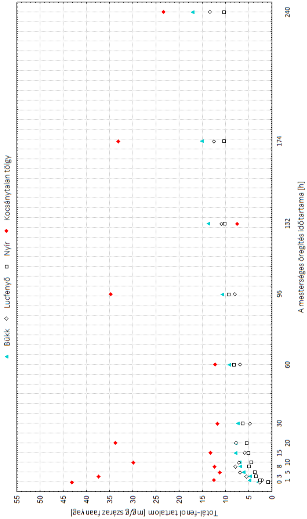
18. ábra A total-fenol tartalom változása különböző fajok esetében, mesterséges öregítés (0-240h) hatására (átlagértékek) (0h: kontroll minta)
