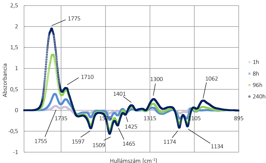
22. ábra Nyír faanyag különbségi színeképei 1, 8, 96 és 240h idejű mesterséges öregítés hatására (ujjlenyomat tartomány, 1900-900 \text{cm}^{-1} )
