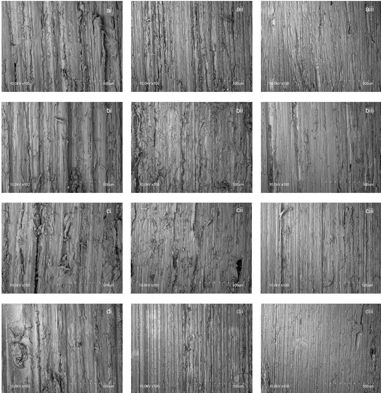
11. ábra Pásztázó elektronmikroszkópos felvételek a meghatározott érdesség tartományokhoz tartozó jellemző csiszolószemcse finomságú csiszolópapírral csiszolt felületeken
