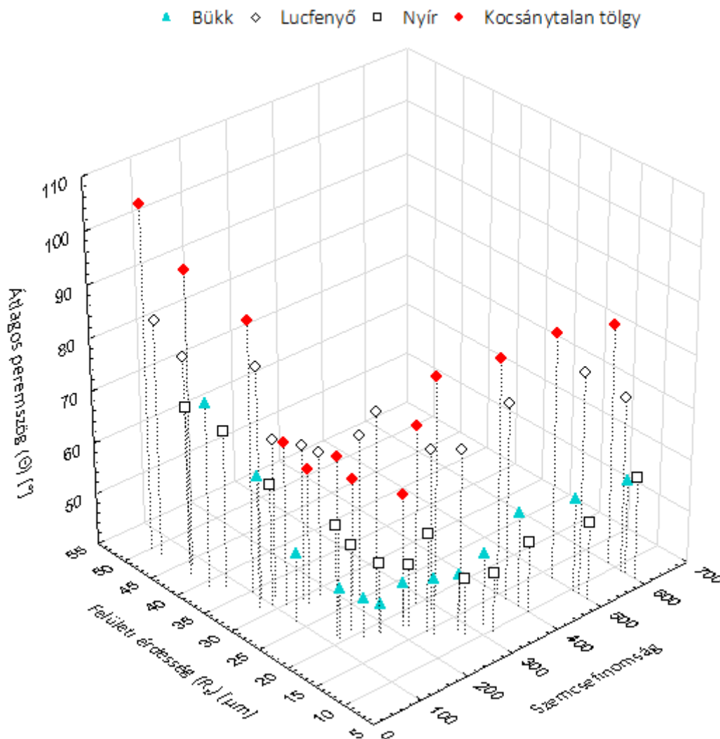
9. ábra Csiszolt fafelületeken mért átlagos peremszög értékek, az átlagos egyenetlenség magasság ( R_z ) és szemcsefinomság függvényében
