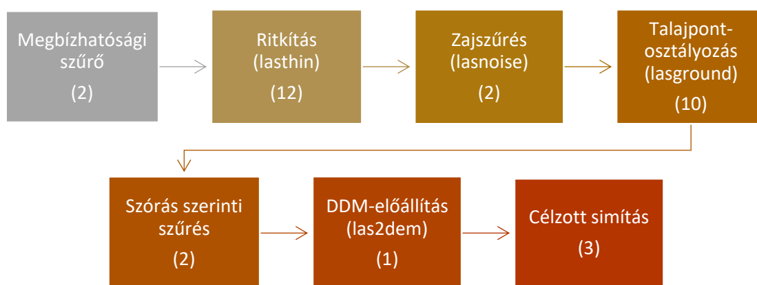
20. ábra: Domborzatmodellek előállításának lépései, az egyes lépések lehetséges paraméterszámával
