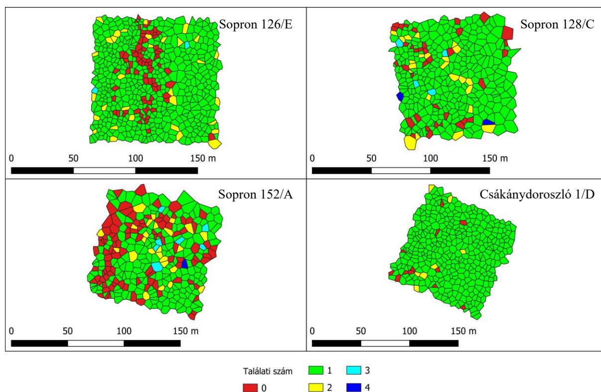
39. ábra: A faegyedek Voronoi-poligonjaira eső találási számok
