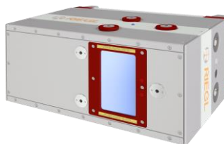
26. ábra: Riegl VQ780 II szenzor (forrás: rieg.com)
