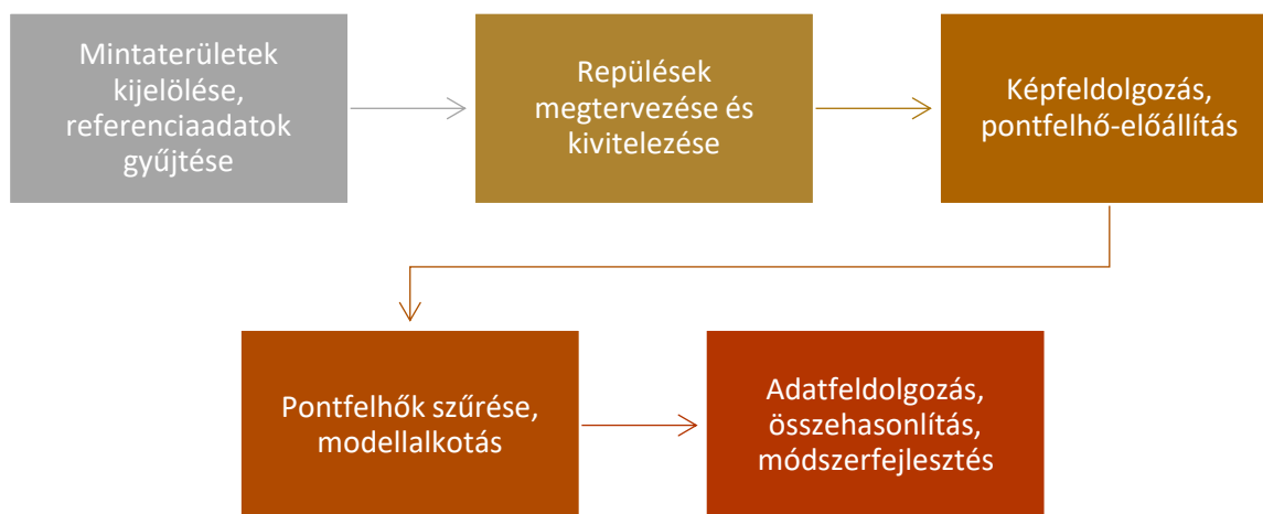
9. ábra: A módszerek kidolgozásának fő lépései
