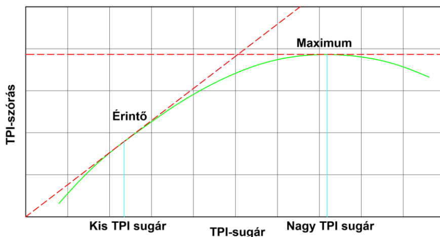
27. ábra: A TPI-sugarak megválasztását elősegítő modell
